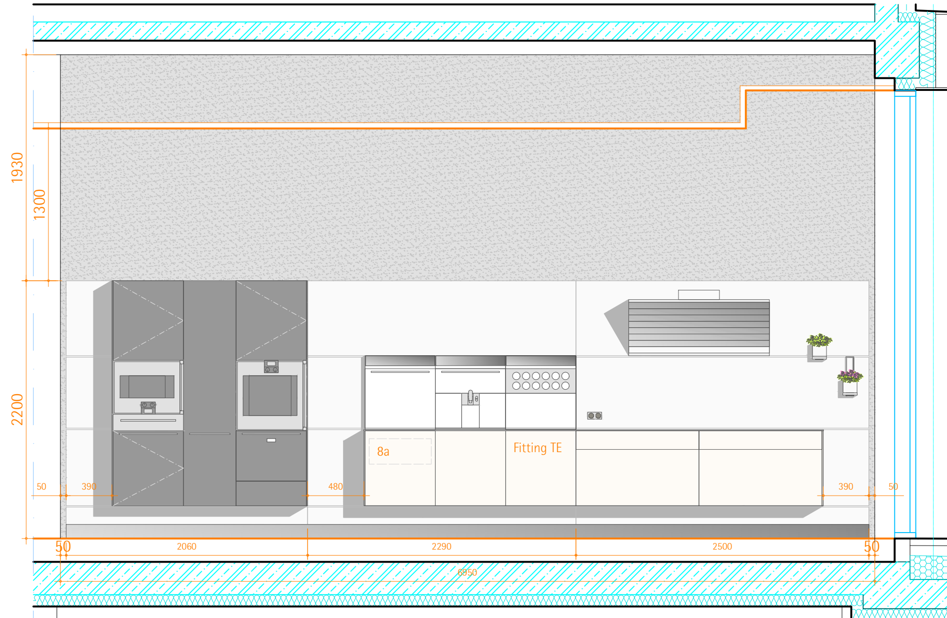
Elevation A
