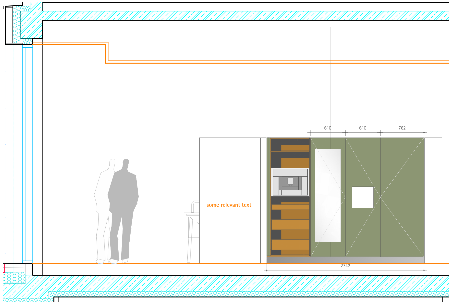
Elevation E
