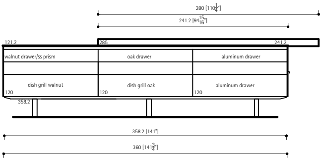
ELEVATION A
